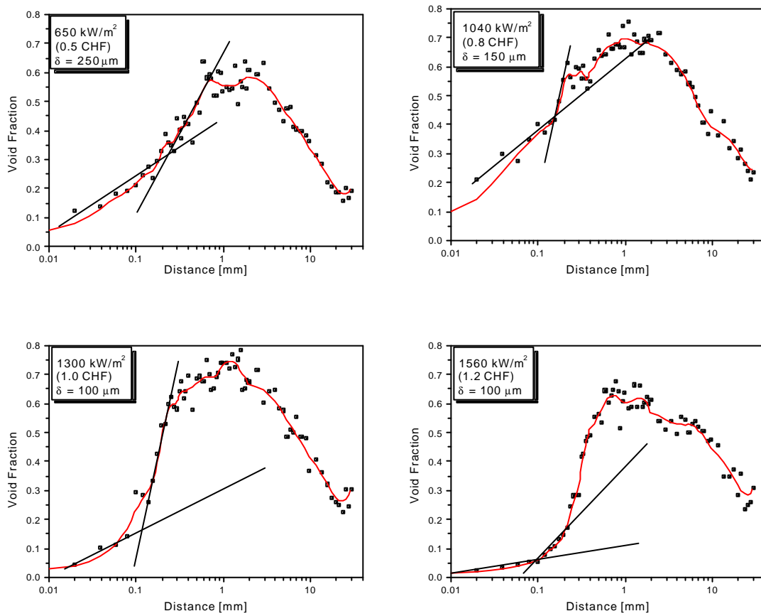
Fig. 6 Void fraction distribution ( D=30 \text{ mm} )
