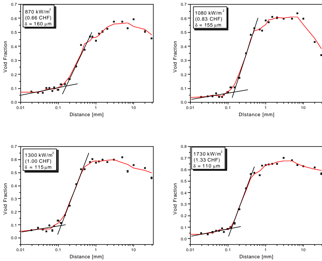
Fig. 5 Void fraction distribution (D=25 mm)
