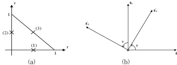
그림 1. (a) 3절점 판 유한요소의 전단변형률장을 형성하기 위한 공변(covariant)변형률을 구하는 지점(tying points); (b) \theta 회전된 공변기저벡터( g'_r , g'_s )와 회전 전 공변기저벡터( g_r , g_s ).
