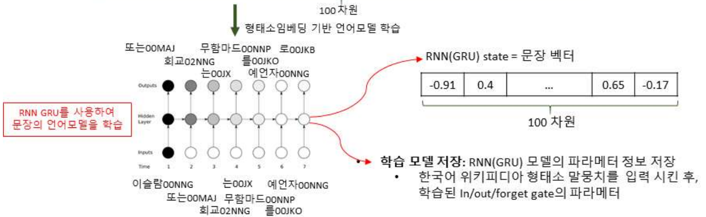
그림 3 형태소임베딩 모델 기반 한국어 문장 언어모델 학습 과정
