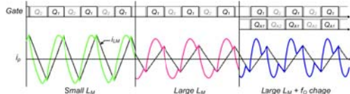
그림 4 L_M 값과 f_o 변경에 따른 1차 측 전류 파형
