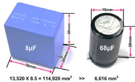
그림 1 필름 캐패시터와 전해 캐패시터 크기 비교(450V/68µF)
