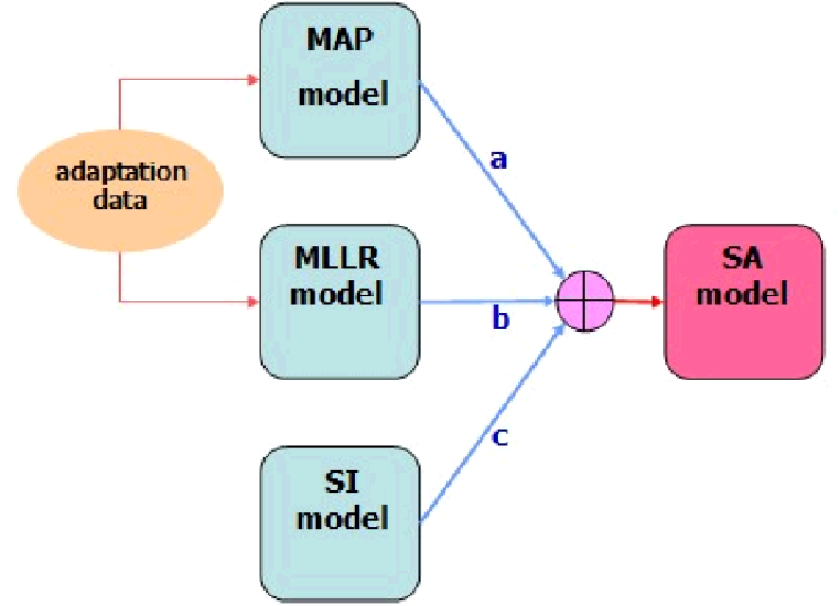
[그림 1] hybrid speaker adaptation
