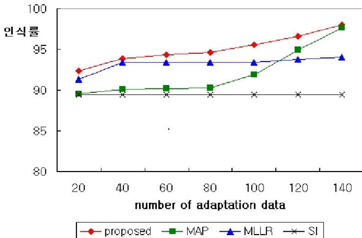
[그림 2] 인식 성능 비교
