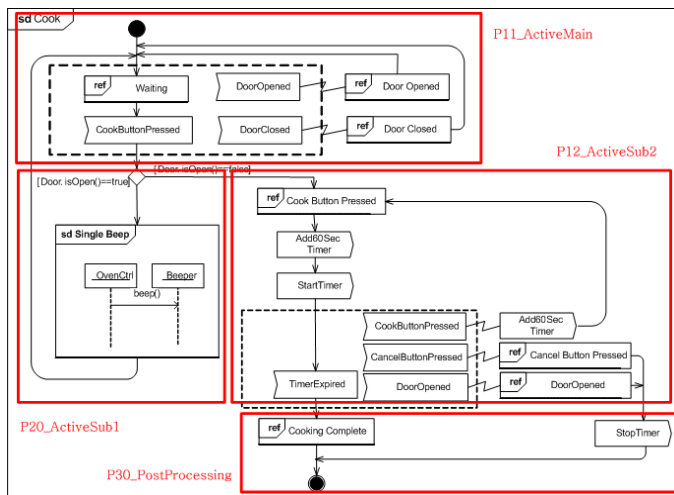
그림 4. ESUML: 소프트웨어 물리적 모델
