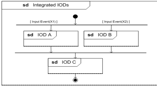
그림 3. IOD 통합에 의한 광역행위 표현
