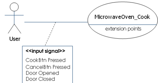
<그림 2> Use Case 모델링 예제
