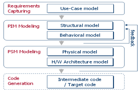
<그림 1> ESUML 모델링 절차
