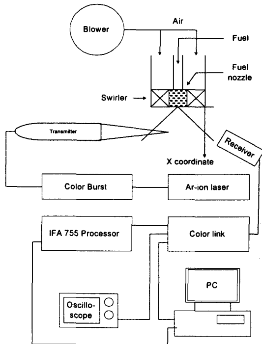
Fig. 2 APV setup
