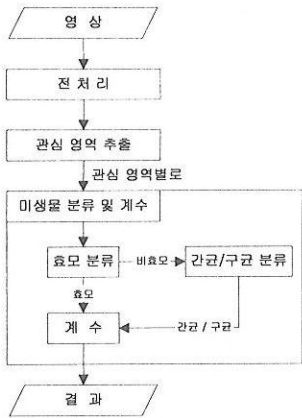
그림 2. 시스템의 흐름도
