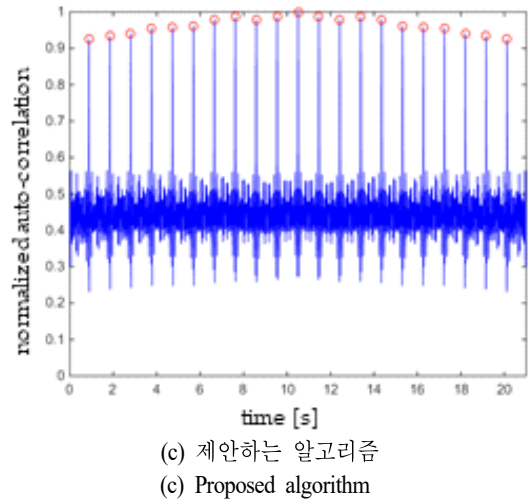
그림 7. Spool peak 탐지 결과 - 모델 A Fig. 7. Results of spool peak detection - model A.
