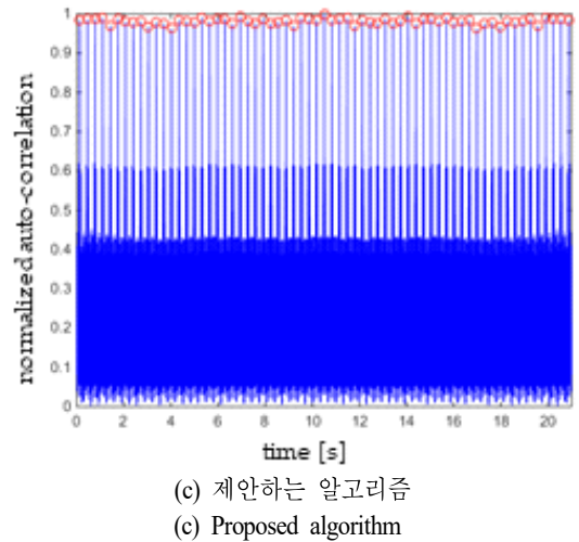
그림 8. Spool peak 탐지 결과 - 모델 B Fig. 8. Results of spool peak detection - model B.
